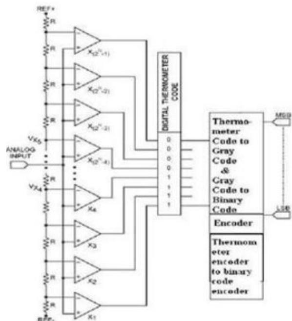
Fig.1. Flash ADC Block Diagram.
